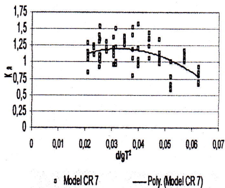
Gambar 4.7 Grafik hubungan K_a terhadap d/gT^2 pada model CR- 7
