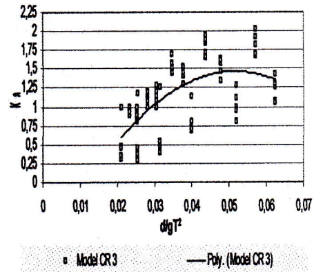
Gambar 4.3 Grafik hubungan K_a terhadap d/gT^2 pada model CR- 3
