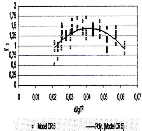
Gambar 4.5 Grafik hubungan K_a terhadap d/gT^2 pada model CR- 5
