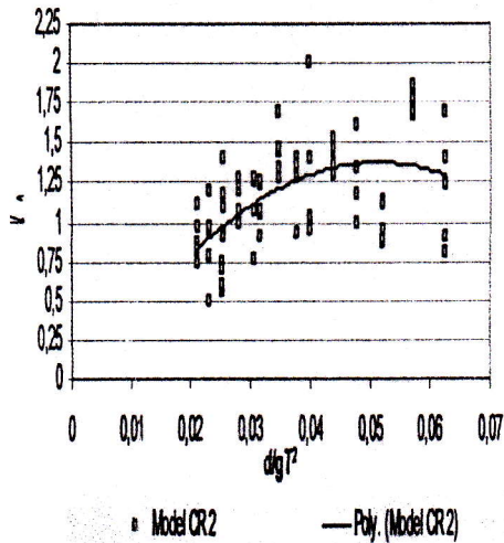
Gambar 4.2 Grafik hubungan K_a terhadap d/gT^2 pada model CR- 2
