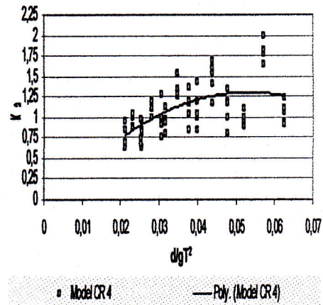
Gambar 4.4 Grafik hubungan K_a terhadap d/gT^2 pada model CR- 4
