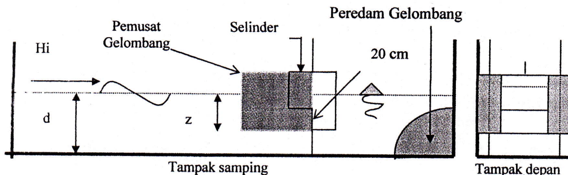
Gambar 3.2 Saluran gelombang dengan model fixed OWC
