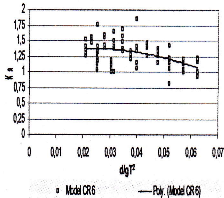
Gambar 4.6 Grafik hubungan K_a terhadap d/gT^2 pada model CR- 6
