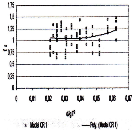
Gambar 4.1 Grafik hubungan K_a terhadap d/gT^2 pada model CR- 1
