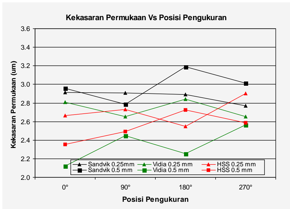
Gambar 8. Grafik Hubungan Kekasaran Permukaan dan Posisi Titik Uji untuk untuk Variasi Material Pahat, Kedalaman Potong dan Feeding
