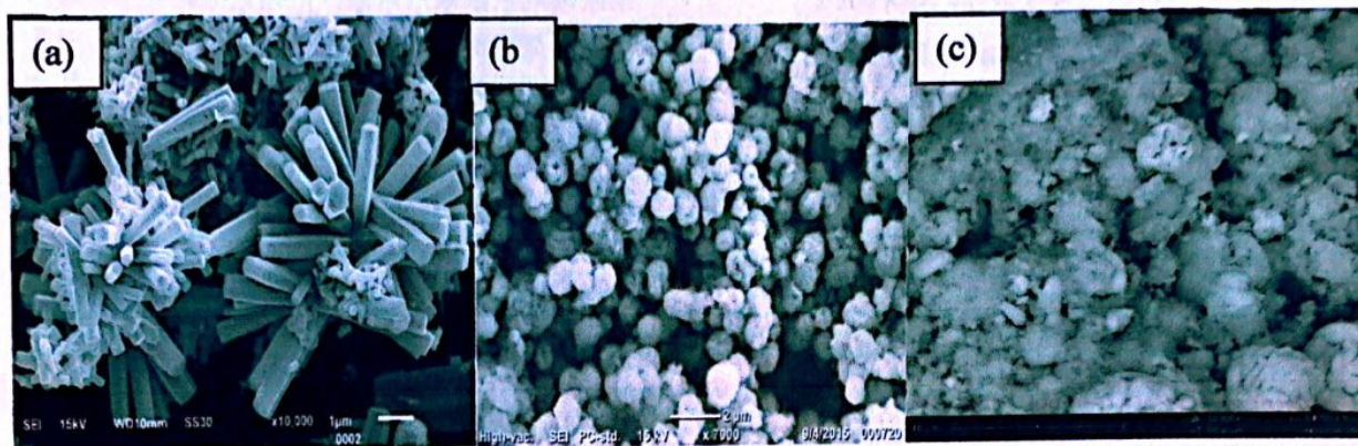
Gambar 2. SEM morfologi nanopartikel ZnO (a). tanpa penambahan ekstrak, (b) dengan penambahan ekstrak air Hibiscus rosa sinensis , (c). dengan penambahan ekstrak air Allium sativum
