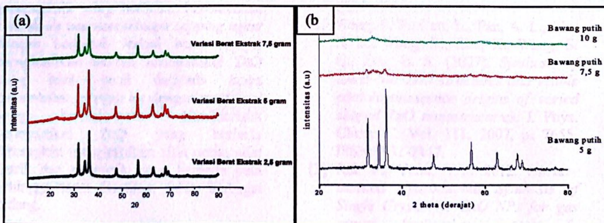
Gambar 1. Difraktogram ZnO dengan penambahan ekstrak air tanaman pada berbagai variasi berat sampel (a). Hibiscus rosa sinensis , (b). Allium sativum .
