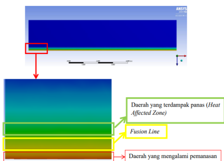
Gambar 17. Hasil Simulasi Fenomena Perpindahan Panas dan Daerah Berdampak Panas pada Sumbu X_0, Y_0 hingga X_{10051}, Y_0
