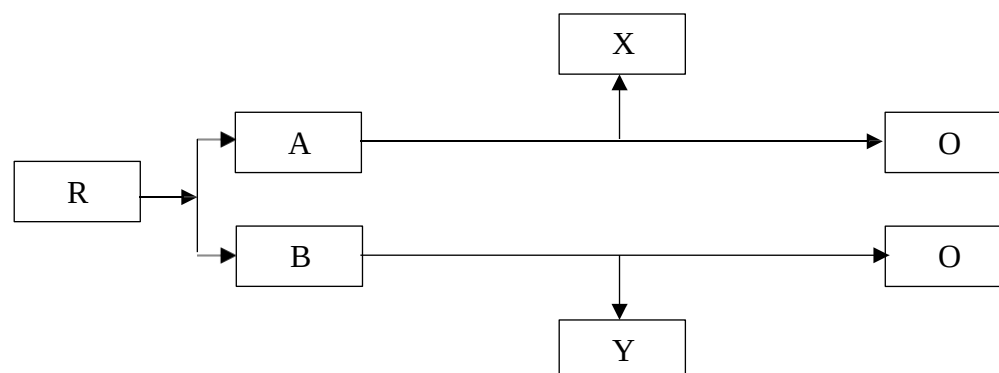
Gambar 4.1. Desain penelitian
